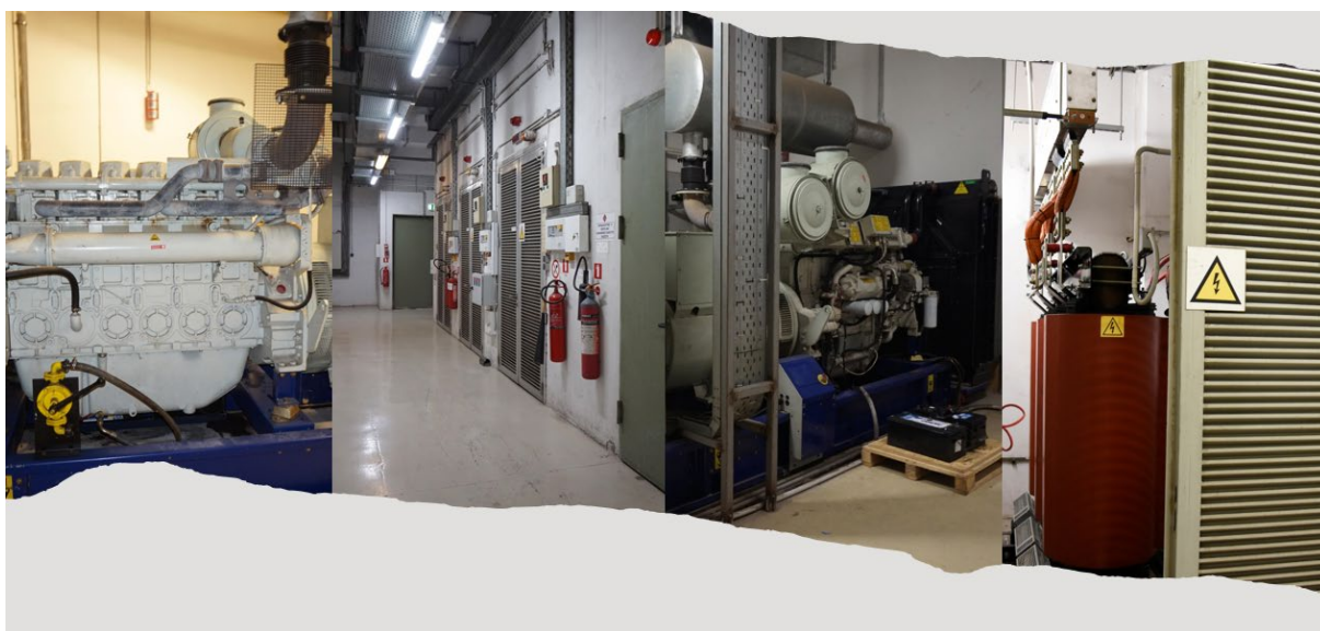
Εικόνα 8: Υποσταθμός μέσης τάσης και εγκαταστάσεις διανομής ενέργειας του Εμπορικού και Ψυχαγωγικού Κέντρου «The Mall Athens»
