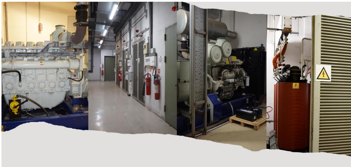
Εικόνα 7: Υποσταθμός μέσης τάσης και εγκαταστάσεις διανομής ενέργειας του Εμπορικού και Ψυχαγωγικού Κέντρου «The Mall Athens»
